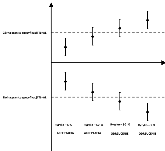
Zasada A. Prostej akceptacji pasmo ochronne w=0
