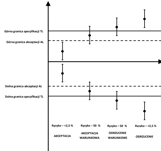
Zasada B . Zasada akceptacji z pasmem ochronnym w=U
